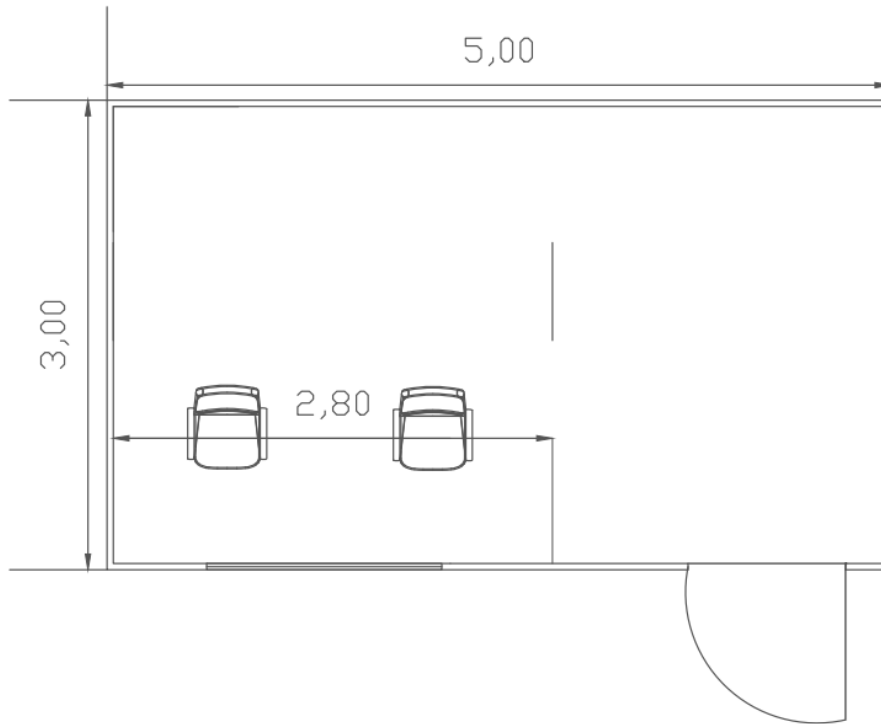
Σχήμα 1. Σκαρίφημα κάτοψης οικίσκου με εξωτερικές διαστάσεις Μ:5,00 x Π:3,00 x Υ: 2,75 -2,85 μέτρα
