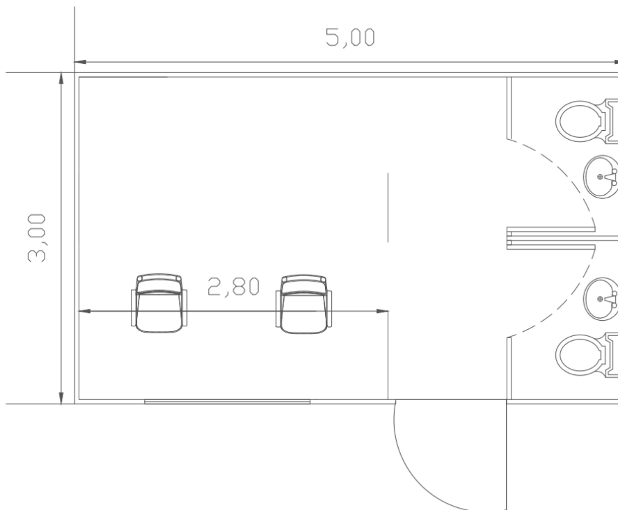
Σχήμα 2. Σκαρίφημα κάτοψης οικίσκου με εσωτερικά WC
